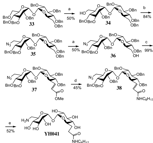
Scheme 8. Reagents: (a) (1) Ac 2 O, TMSOTf; (2) NaOMe, MeOH; (b) (1) Tf 2 O, CH 2 Cl 2 , py., (2) NaN 3 , DMF; (c) (1) (COCl) 2 , DMSO, DIPEA, (2) MeOC(O)CH 2 P(O)(OEt) 2 , NaH, THF; (d) C 8 H 17 NH 2 , AlMe 3 , CH 2 Cl 2 ; (e) H 2 , Pd(OH) 2 /C, MeOH.
