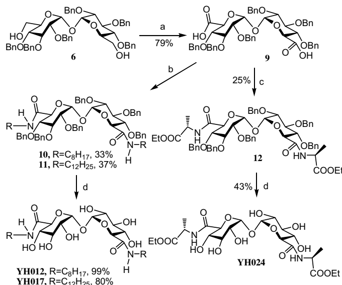
Scheme 3. Reagents: (a) (1) (COCl) 2 , DMSO, DIPEA, (2) NaClO 2 , H 2 O 2 ; (b) (1) (COCl) 2 , (2) C 8 H 17 NH 2 or C 12 H 25 NH 2 ; (c) L-alanine ethylester, EDC, pyr.; (d) H 2 , Pd(OH) 2 /C, MeOH.
